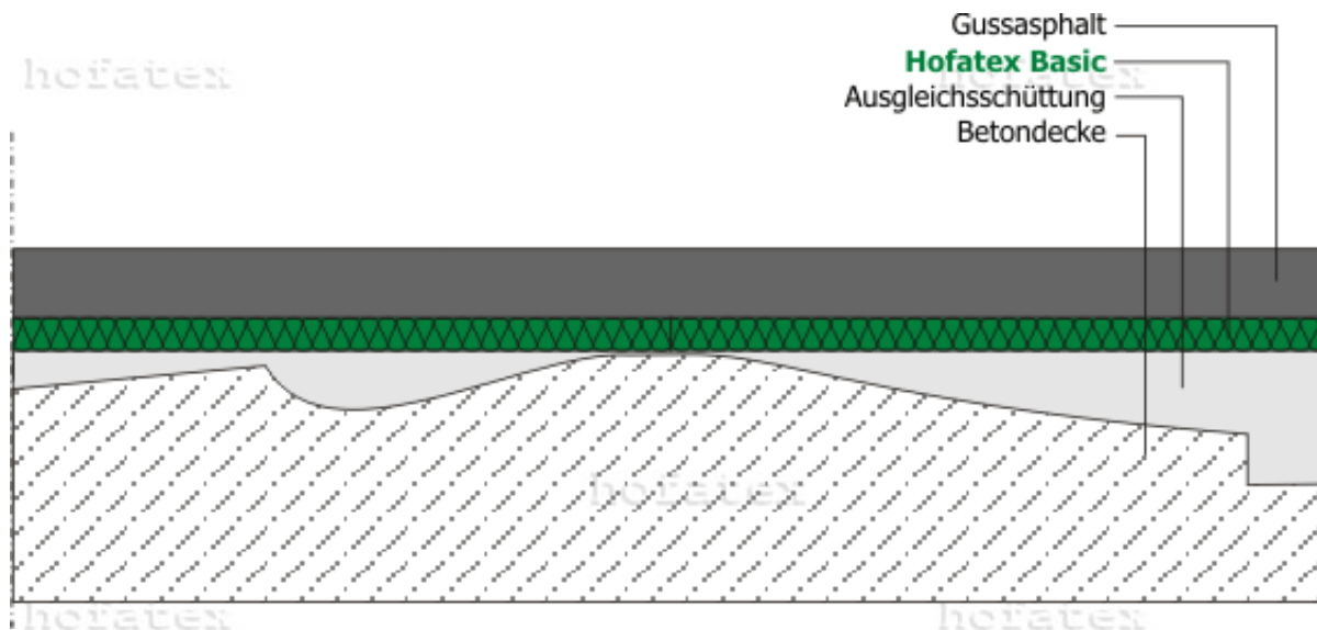
Hofatex Basic auf Ausgleichsschüttung
