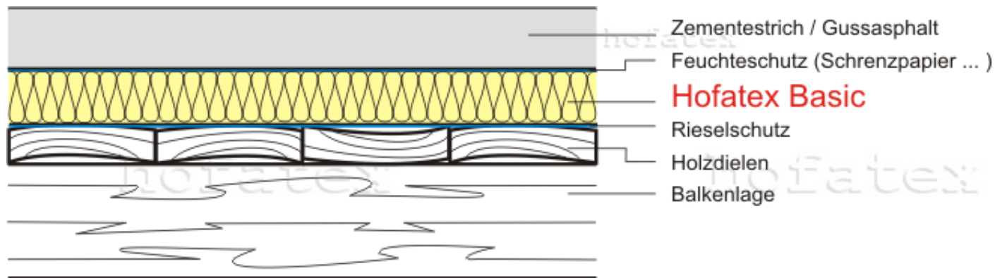
Hofatex Basic auf Holz
