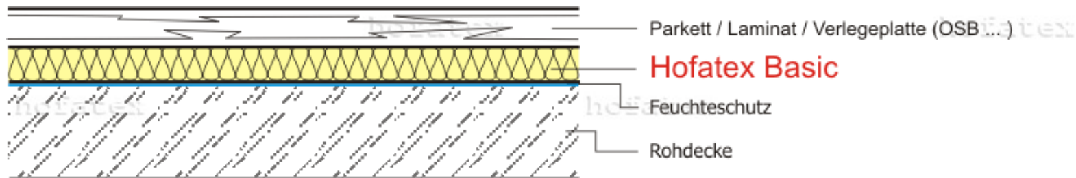
Hofatex Basic auf Beton
